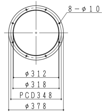
排気接続口フランジ詳細図 (P.V.C製)
