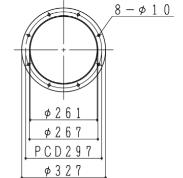
排気接続口フランジ詳細図 (P.V.C製)
