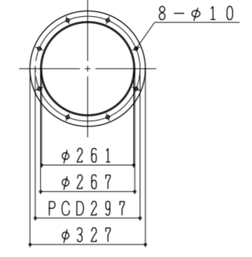
排気接続口フランジ詳細図 (P.V.C製)
